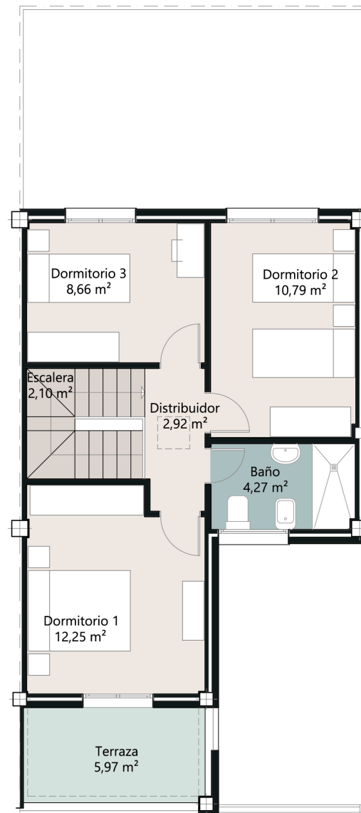
PLANTA PRIMERA
