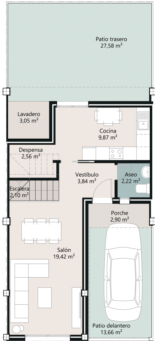
PLANTA BAJA
