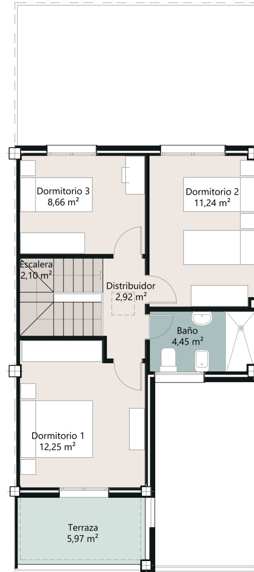
PLANTA PRIMERA
